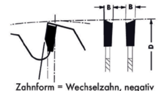
Zahnform = Wechselzahn, negativ
